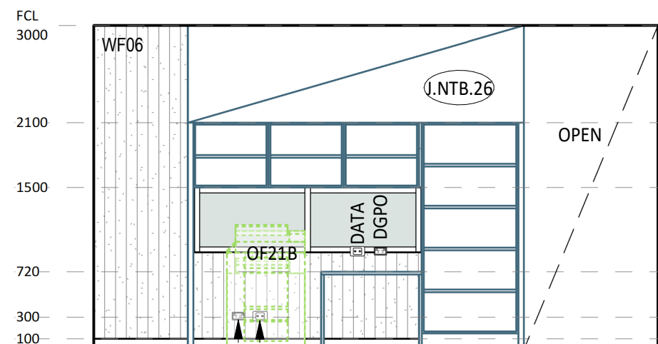
6 ELEVATION DETAIL 60-038 1 : 50
